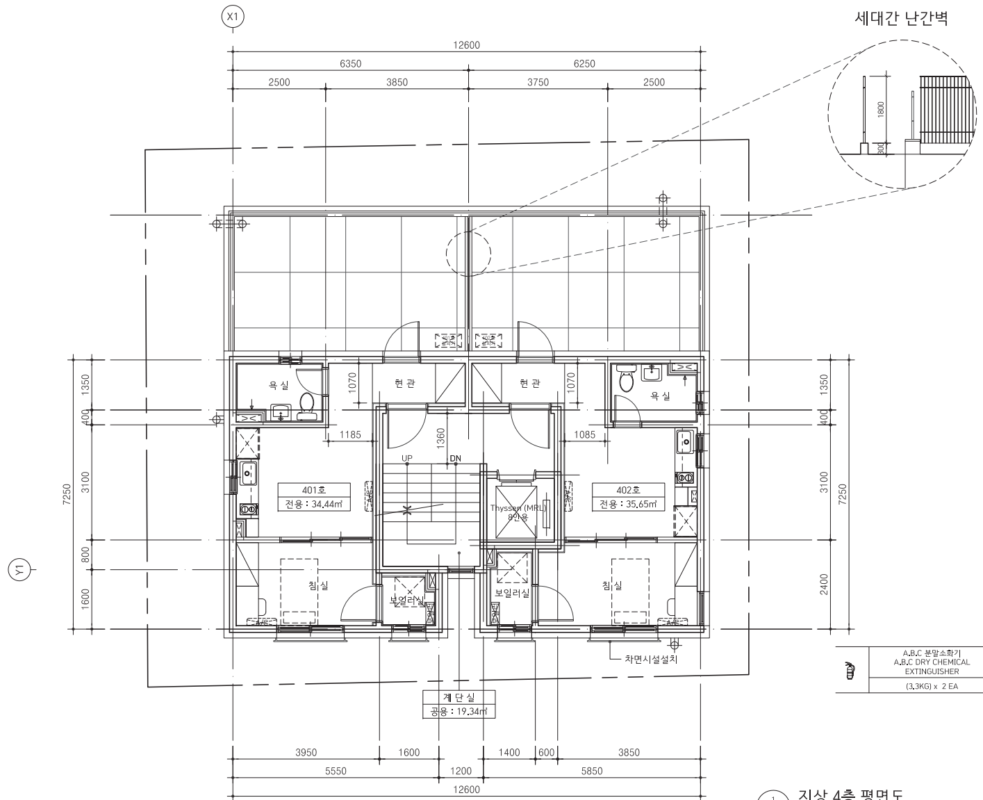
지상 4층 평면도 SCALE : 1/100
