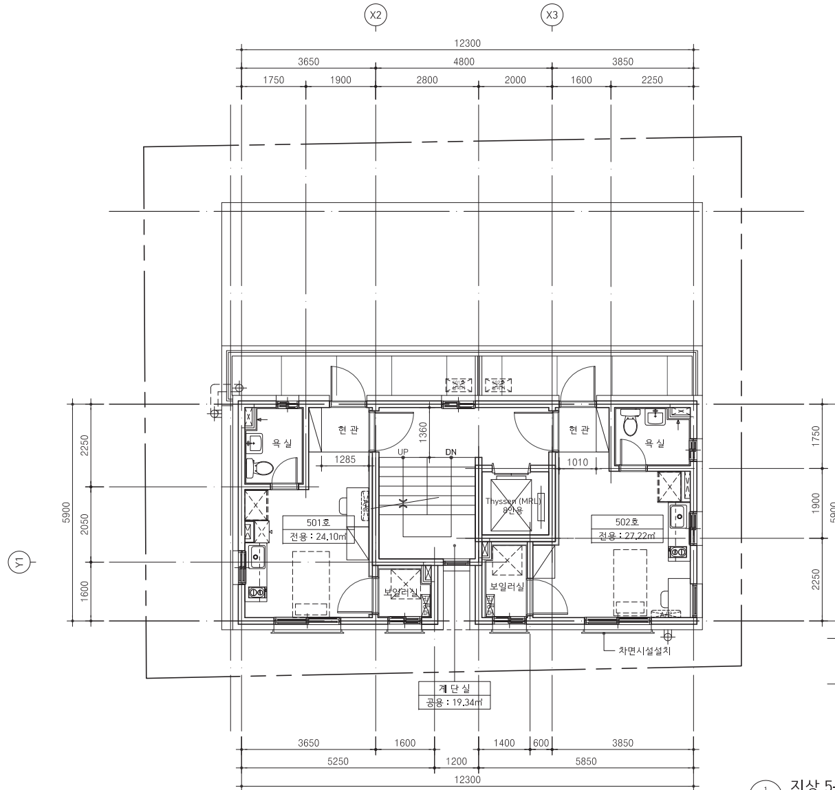
지상 5층 평면도 SCALE : 1/100
