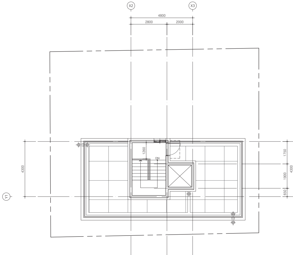
1 옥탑층 평면도 SCALE : 1/100
